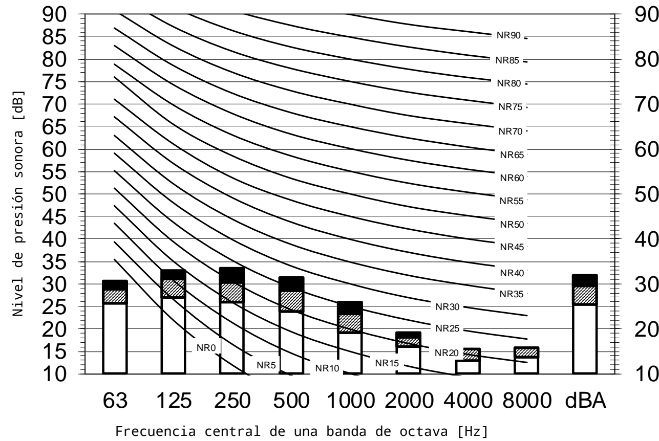
Modo refrigeración
