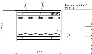
A Vista
