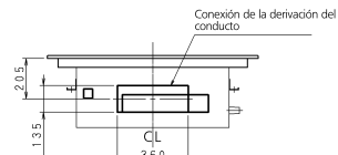
B Vista
