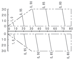
Relación de corrección para capacidad de refrigeración
