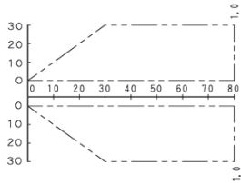
Relación de corrección para capacidad de calefacción
