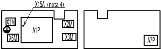
Diseño de la caja de componentes eléctricos
