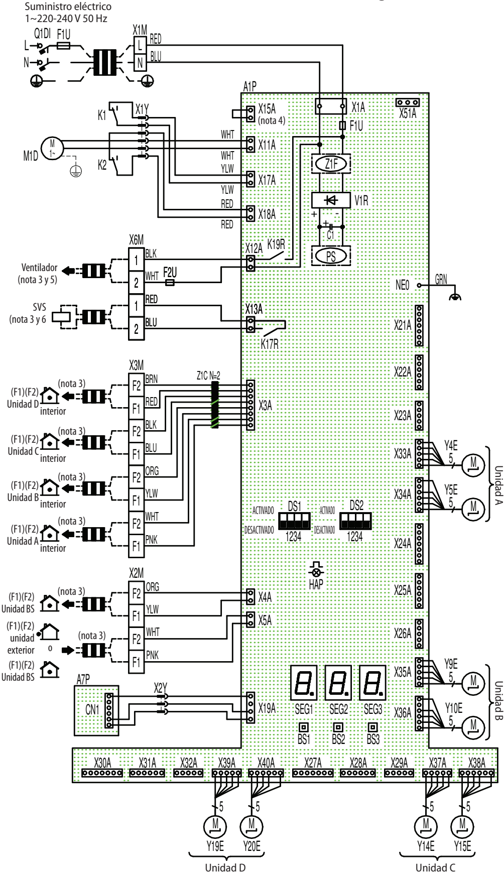
Diseño de la caja de componentes eléctricos
