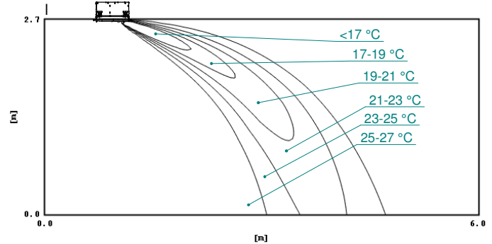
Distribución de temperatura del aire (refrigeración) Sentido de circulación del aire: horizontal
