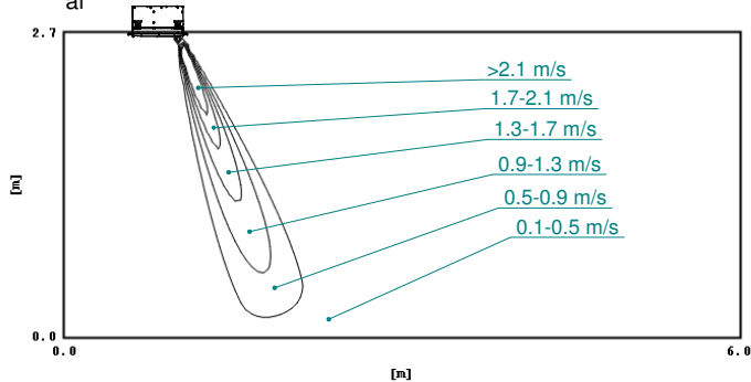
Distribución de velocidad del aire (calefacción) Sentido de circulación del aire: vertical
