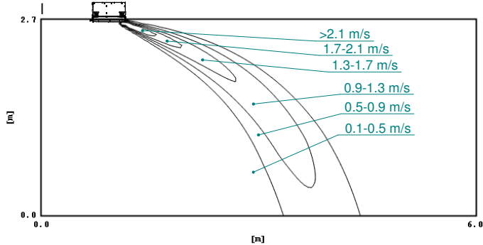
Distribución de velocidad del aire (refrigeración) Sentido de circulación del aire: horizontal
