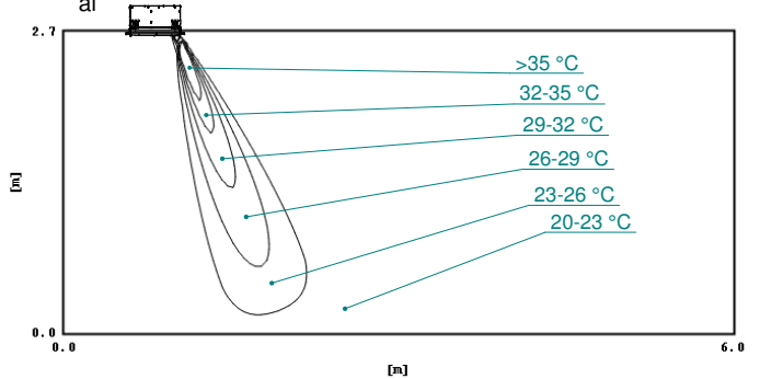
Distribución de temperatura del aire (calefacción) Sentido de circulación del aire: vertical
