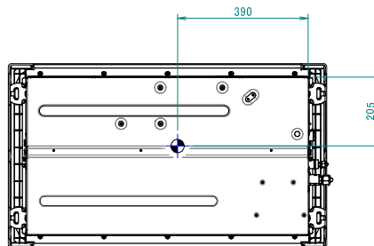
Unidad interior + Panel decorativo
