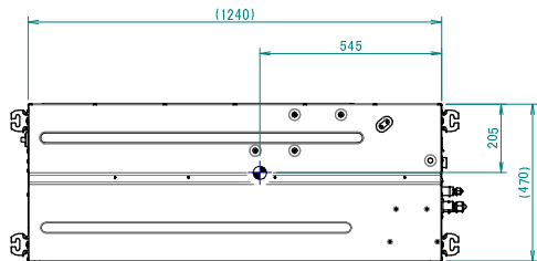
Unidad interior
