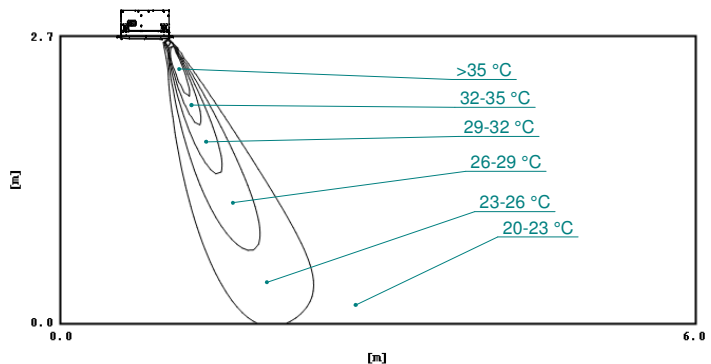
Distribución de temperatura del aire (calefacción) Sentido de circulación del aire: vertical
