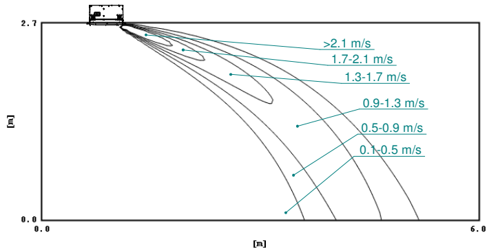
Distribución de velocidad del aire (refrigeración) Sentido de circulación del aire: horizontal
