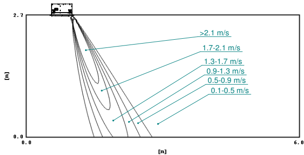
Distribución de velocidad del aire (calefacción) Sentido de circulación del aire: vertical
