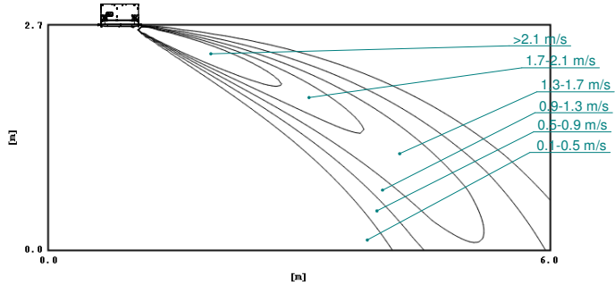
Distribución de velocidad del aire (refrigeración) Sentido de circulación del aire: horizontal
