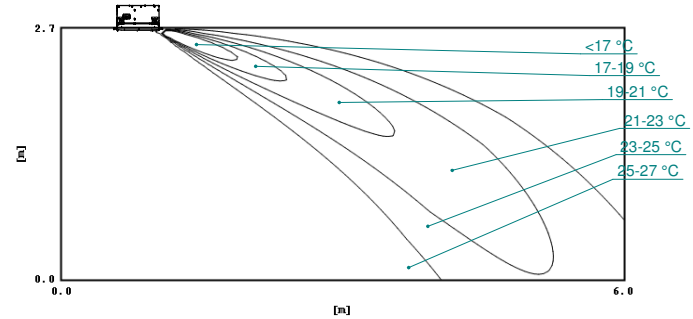
Distribución de temperatura del aire (refrigeración) Sentido de circulación del aire: horizontal
