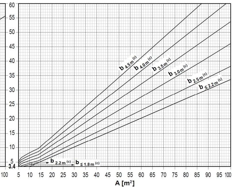
Planta subterránea más baja (b)
