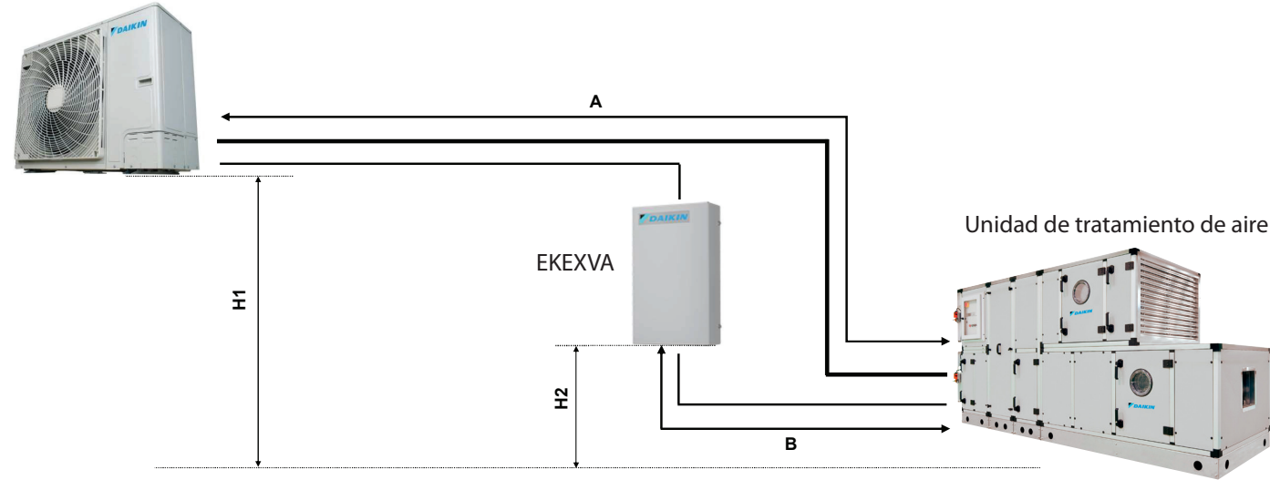
Unidad exterior
