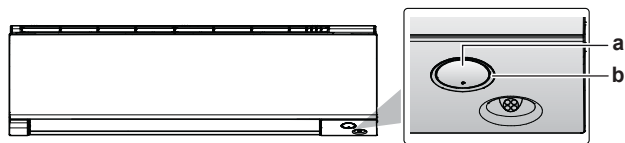
a Daikin Eye b Interruptor de ON/OFF de la unidad interior
