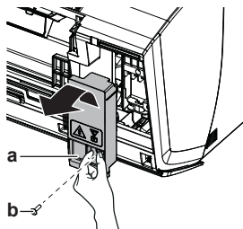
a Tapa de servicio
