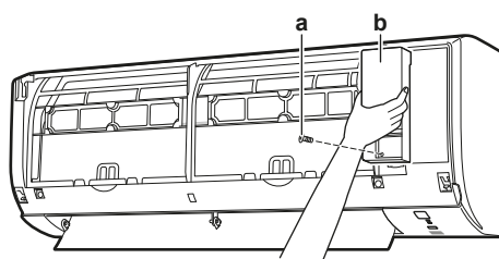
a Tornillo de la tapa de servicio
