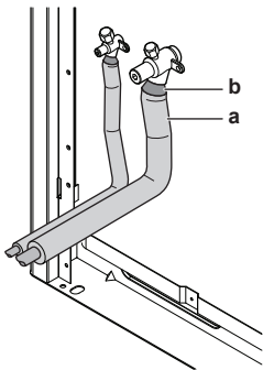
a Material de aislamiento
