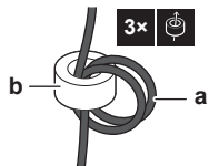
a Cable de interconexión b Núcleo de ferrita
