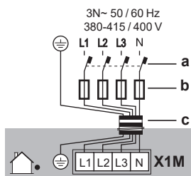
a Disyuntor de fugas a tierra b Fusible c Cable de suministro eléctrico
