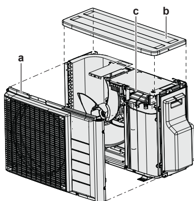
a Placa delantera b Placa superior c Conector S99
