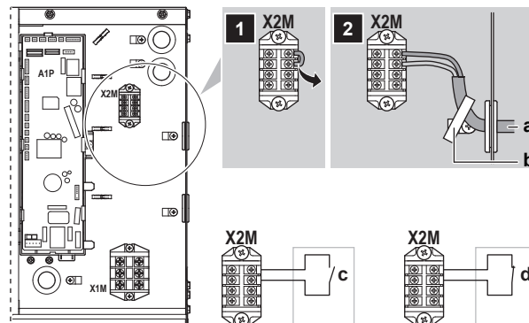
a Contacto de retroalimentación desde la bomba de drenaje b Sujetacables c Fallo de funcionamiento de la bomba de drenaje: Si el contacto se abre, la bomba de calor deja de funcionar y genera un error. d Funcionamiento normal de la bomba de drenaje: Si el contacto se cierra, la bomba de calor reanuda su funcionamiento normal.
