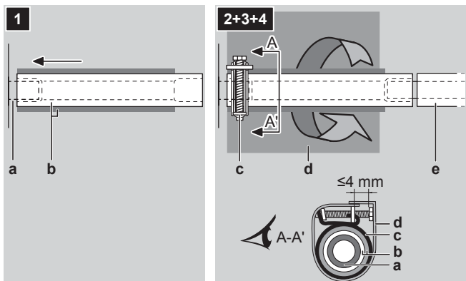
a Conexión de la tubería de drenaje (fijada a la unidad) b Manguera de drenaje (accesorio) c Abrazadera metálica (accesorio) d Almohadilla de sellado (accesorio) e Tubería de drenaje (suministro independiente)
