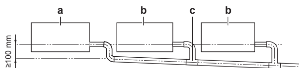
a Unidad del intercambiador de calor b Unidad interior c Junta en T
