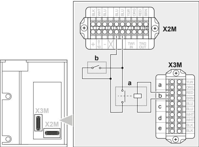
a Relé (normalmente cerrado) (suministro independiente) b Interruptor de caudal (suministro independiente)
