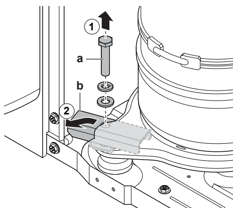
a Perno b Fijador de transporte
