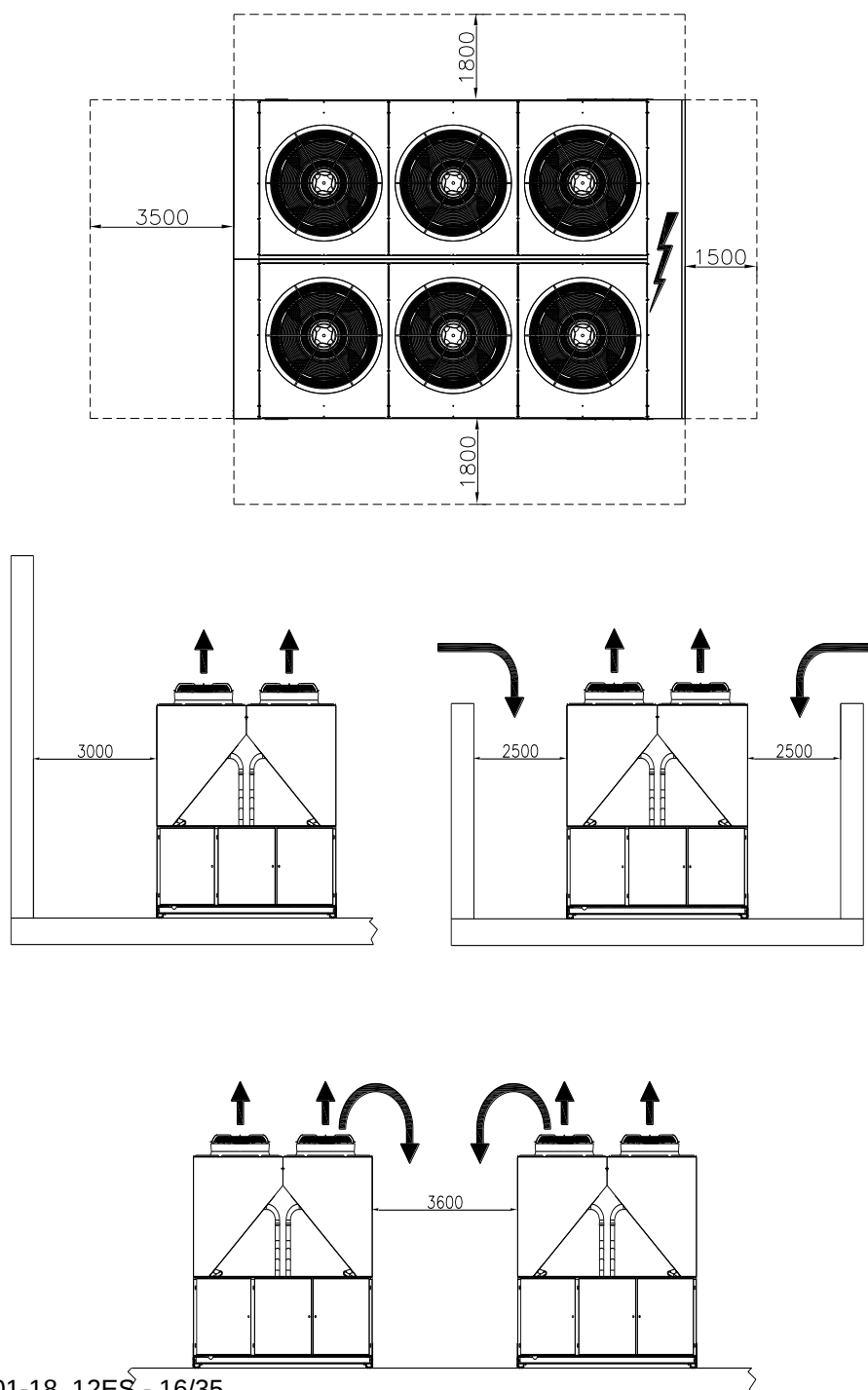
Fig. 5 - Requisitos mínimos de espacio para el mantenimiento de la máquina
