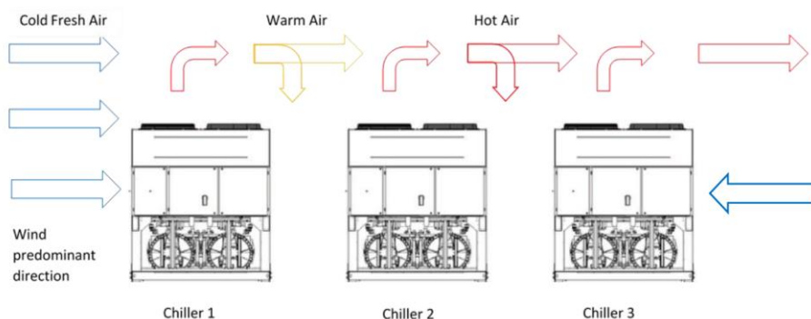
Fig. 6 – Instalación de refrigeradores múltiples
