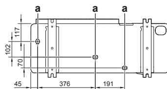
a Orificios de drenaje
