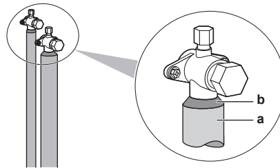
a Material de aislamiento b Calafateado, etc.
