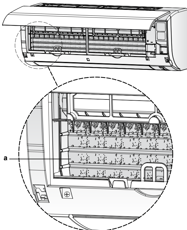
a Placa de blindaje
