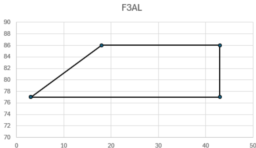
Nueva porción de límite de funcionamiento para compresor F3AL
