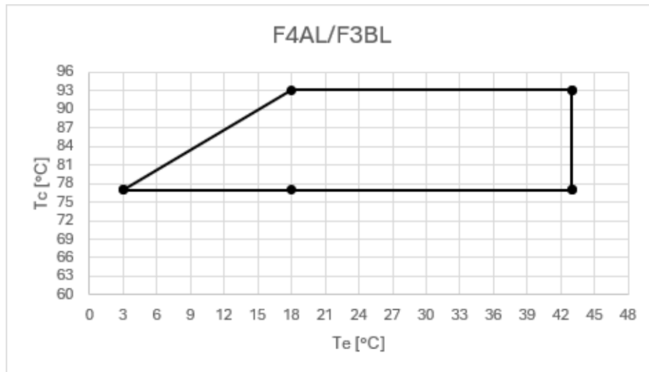
Nueva porción de límite de funcionamiento para compresor F4AL/F3BL
